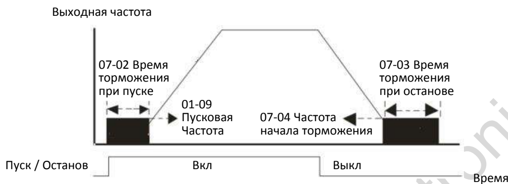
Временная диаграмма торможения постоянным током
